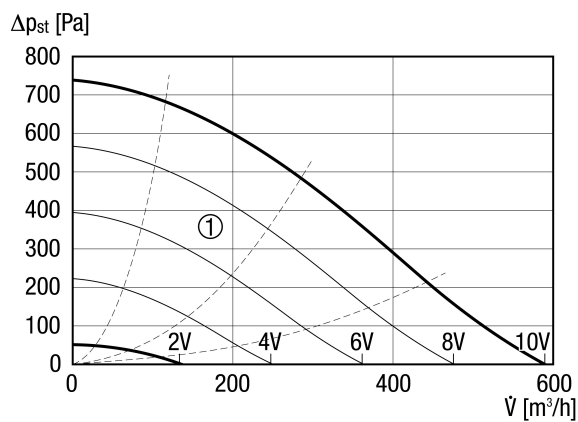
Pomocné charakteristiky pro řízení 2 - 10 V
