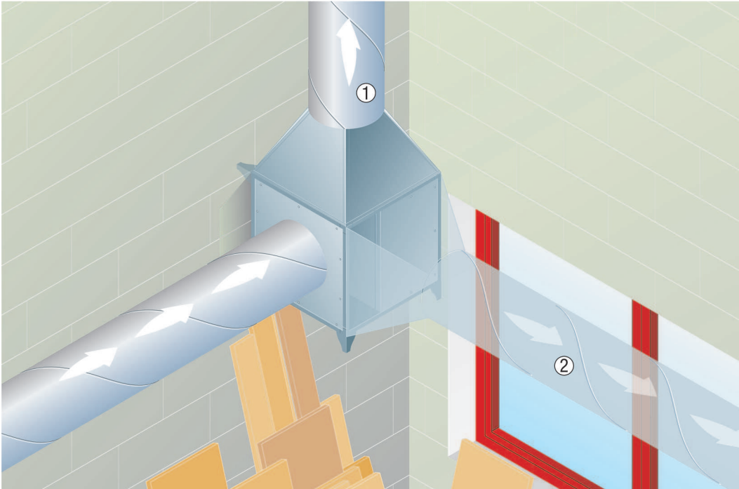
1 - 2 Variable Einbaurichtungen
