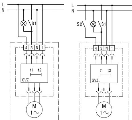
Standardschaltung
