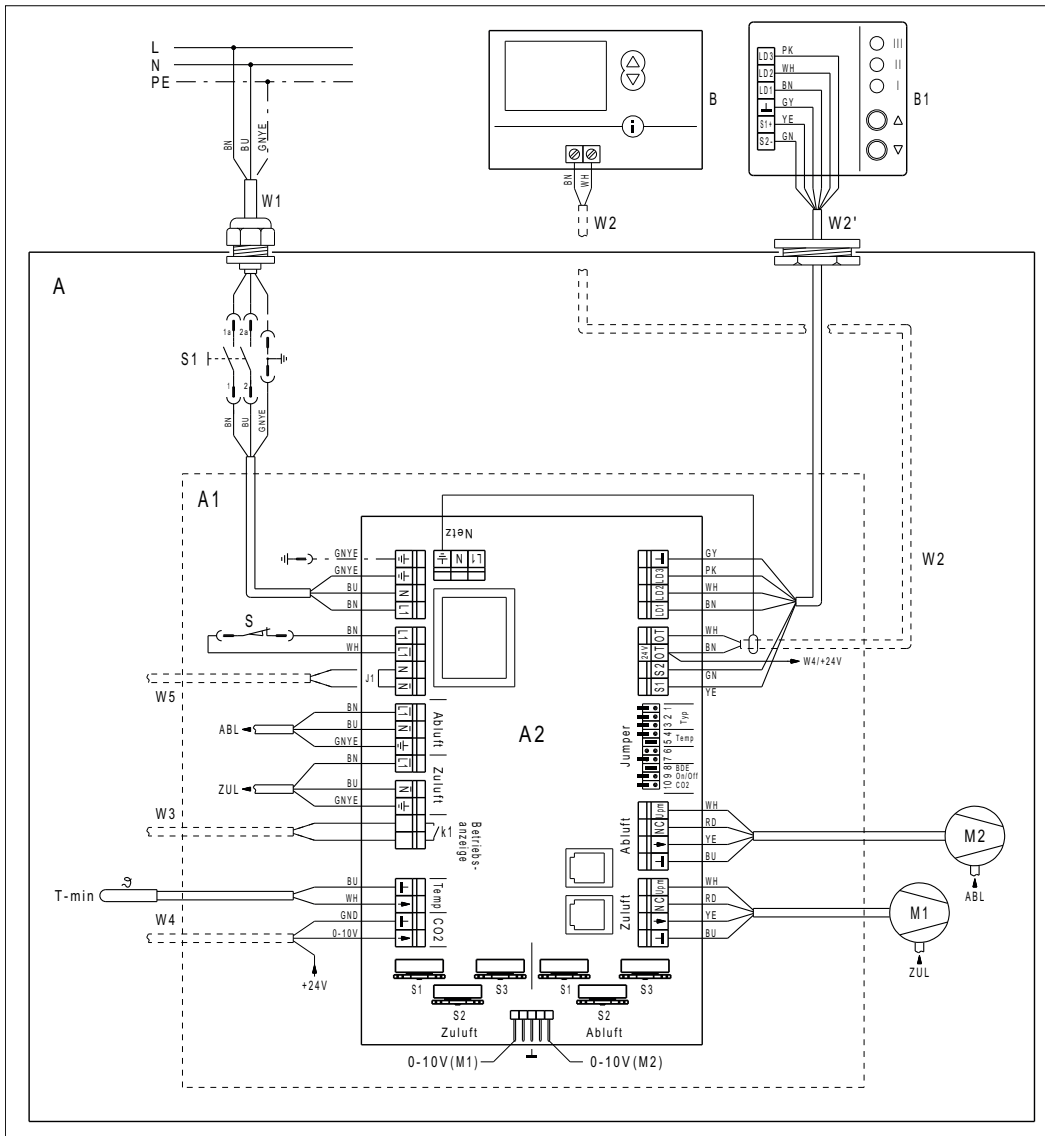
Plan de câblage WS 170 R et WS 170 L
