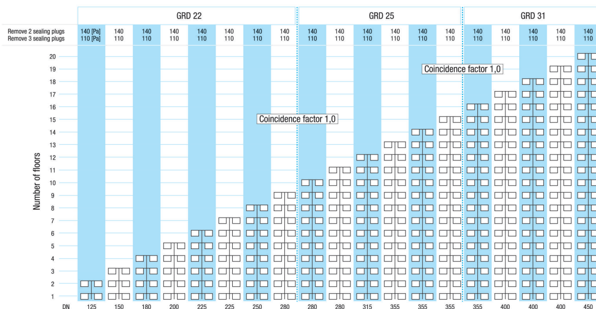
Dijagram 2: Izvedbena shema za odvojeke s dva odsisna elementa po etaži
