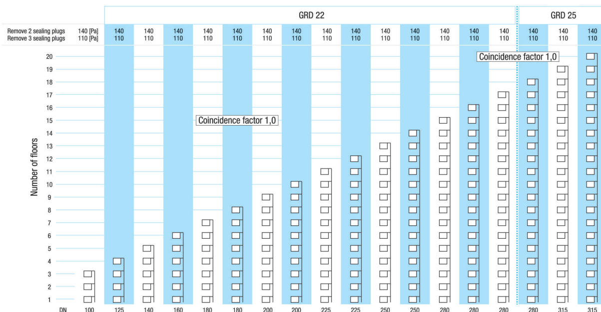
Dijagram 1: Izvedbena shema za odvojeke s jednim odsisnim elementom po etaži
