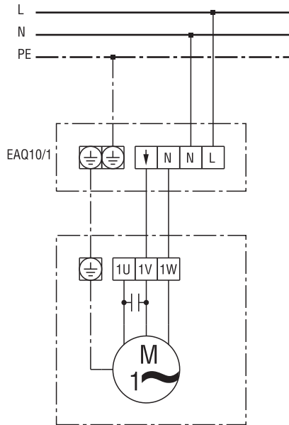
M1 - ventilátor (jobbraforgás)
