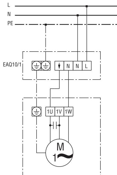
M1 - ventilátor (balraforgás)
