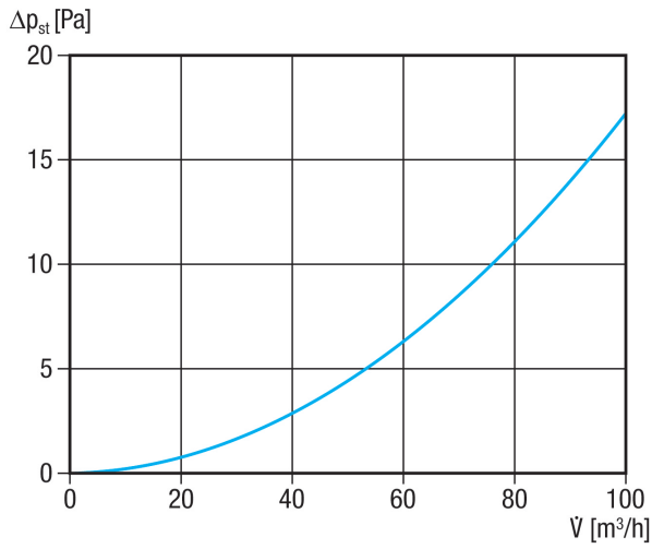
① MF-WL125 80/200 w połączeniu z MF-WE75
